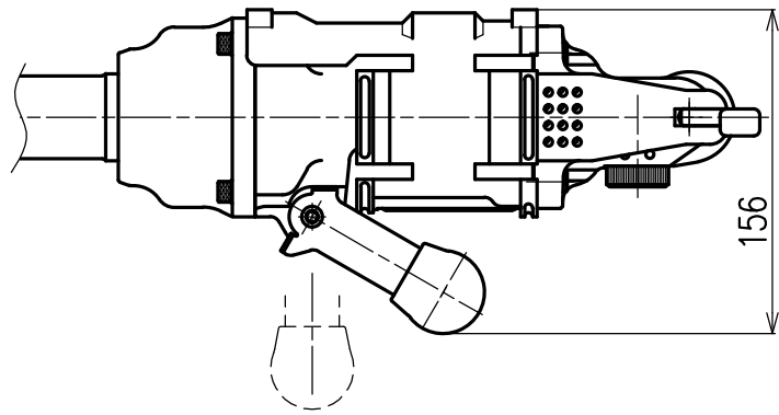
A矢视图 (Dハンドル収納時)
