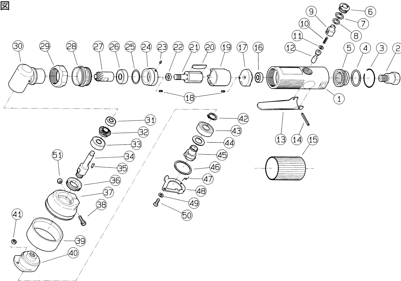
● バランスウエイトC.P構成パーツ
