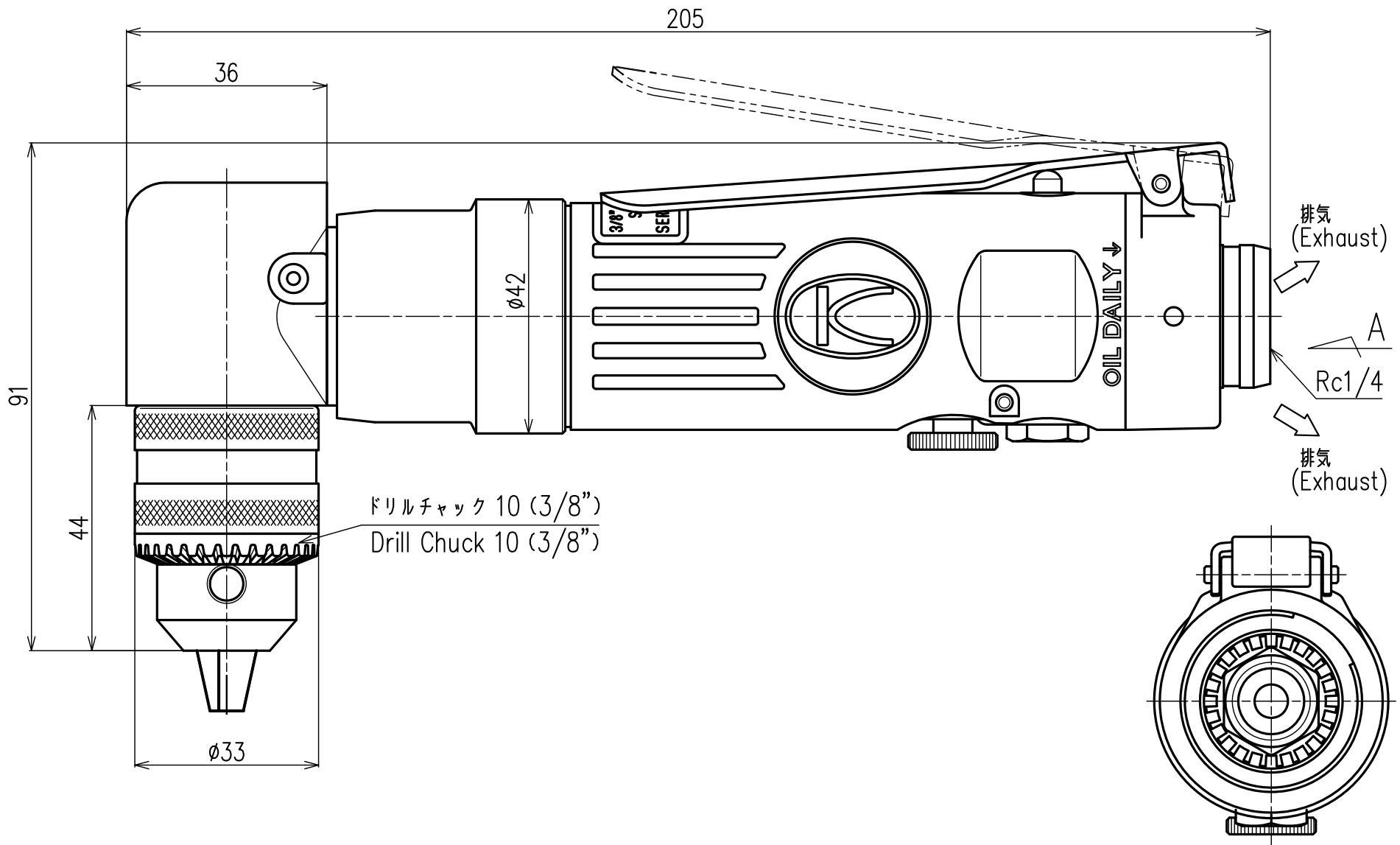
A矢视图
