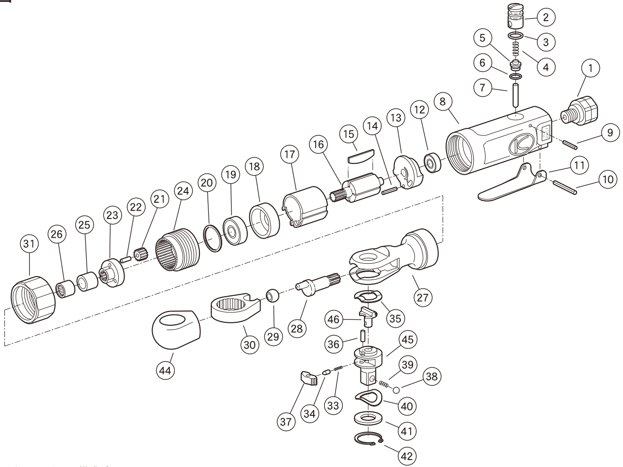
○ ラチェットシャンクC.P構成パーツ
