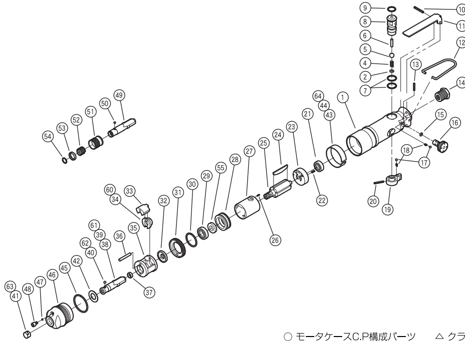
○ モーターケースC.P構成パーツ △ クラッチケースC.P構成パーツ
